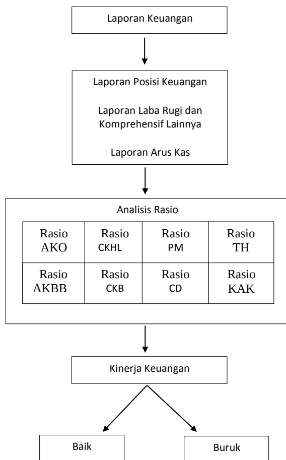
Gambar 2.1 Kerangka Konseptual
