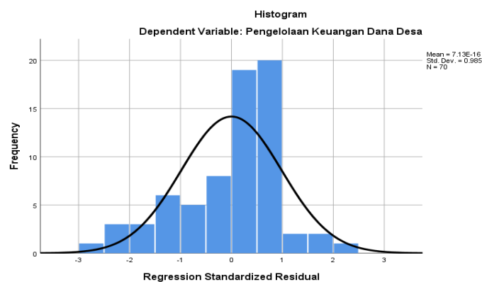
Gambar 4.2 Grafik Histogram
